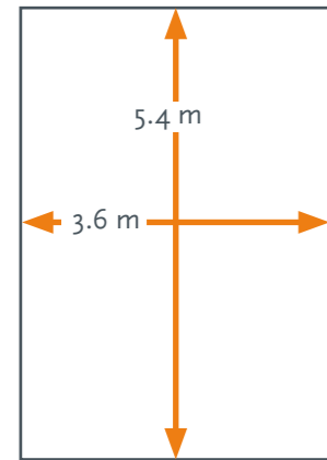
Afmetingen standaardkantoorunit
